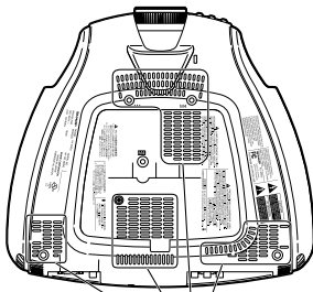
Einlass-Lüftungsöffnungen.
